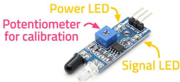
Fig 4: IR Module
