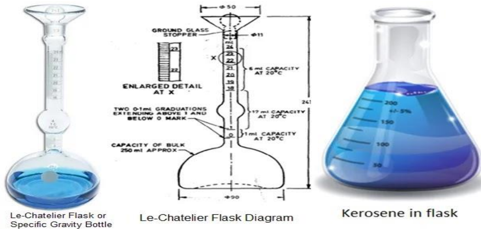
Fig: 2. 6. Le-Chatelier Flask
