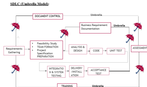
Fig 1: SDLC (Umbrella Model)
