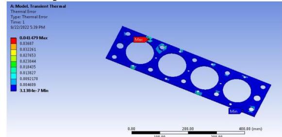
Fig 15: Thermal Error
