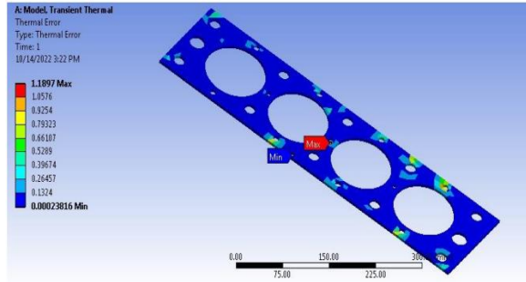
Fig 22: Thermal Error
