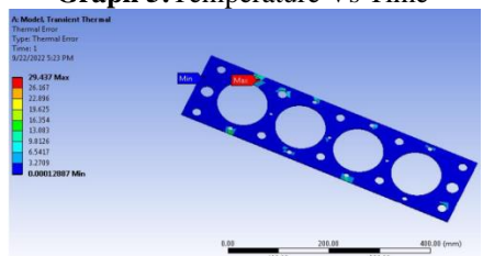
Fig 8: Thermal Error
